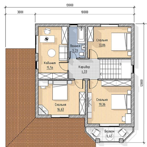
План 1 этаж
