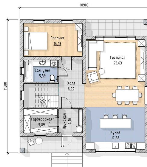
План 1 этаж
