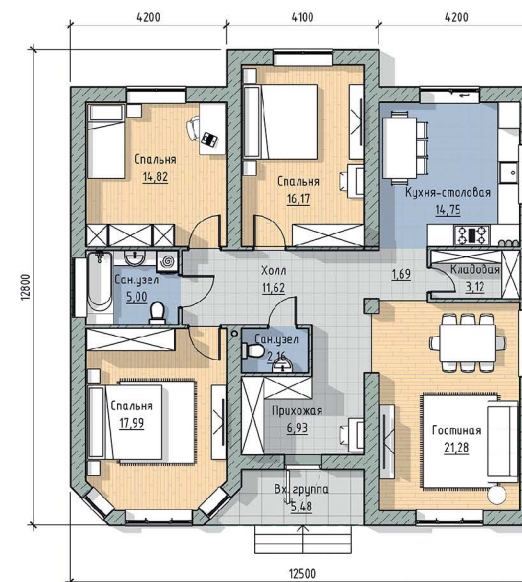
План
