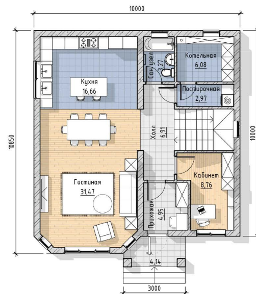
План 1 этаж
