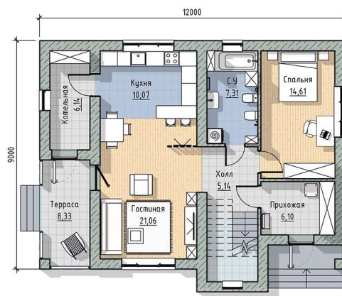
План 1 этаж
