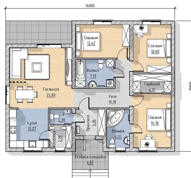
План
