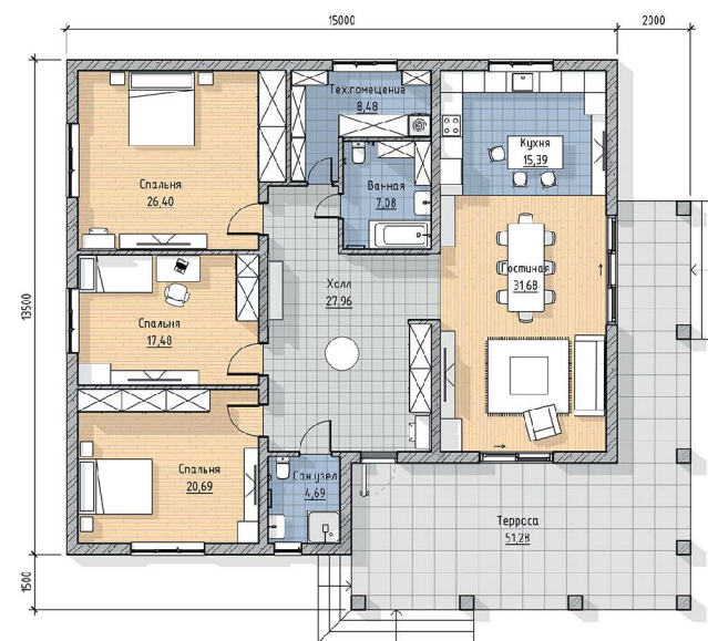
План
