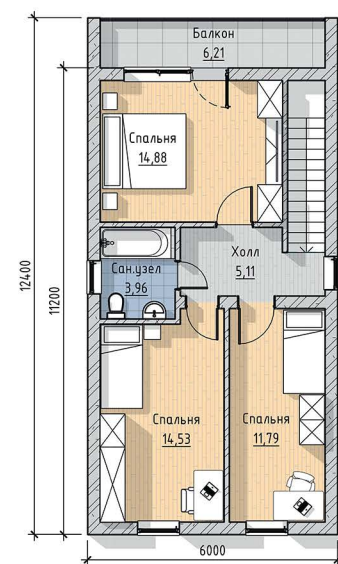
План 2 этаж
