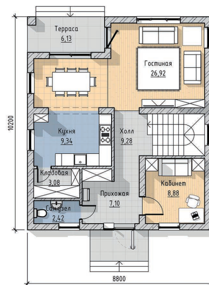
План 1 этаж
