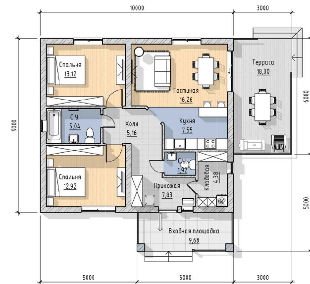
План
