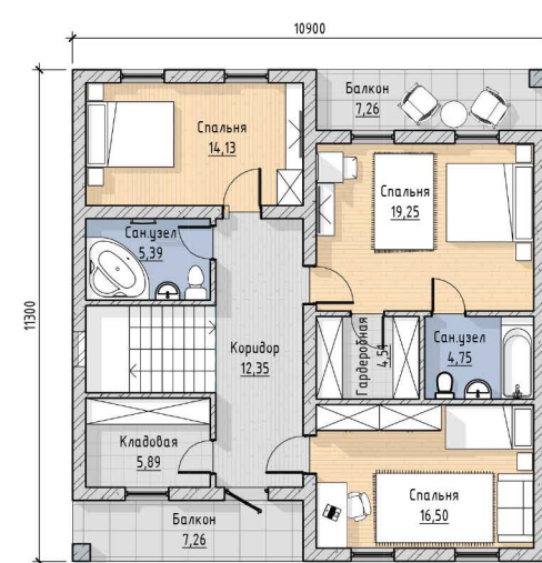
План 2 этаж
