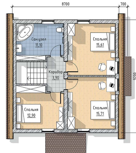
План 2 этаж
