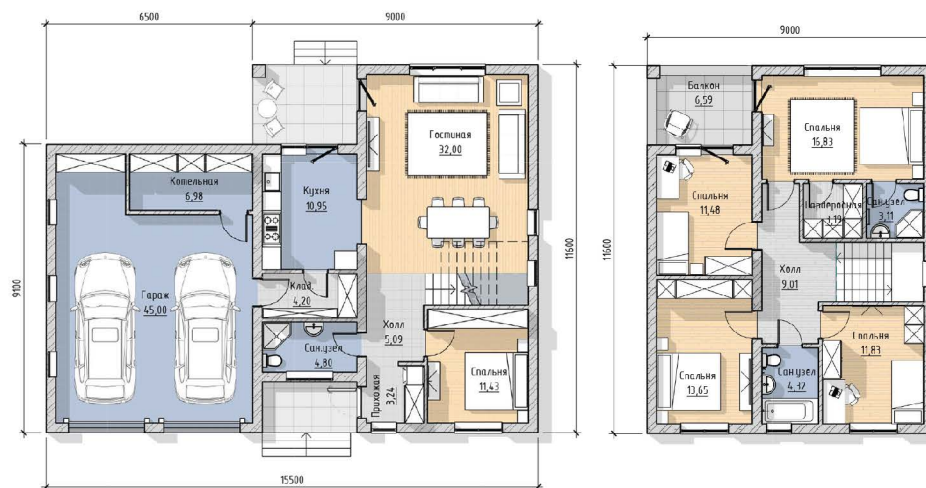
План 1 этаж
