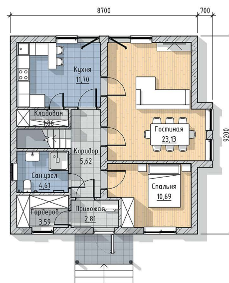
План 1 этаж
