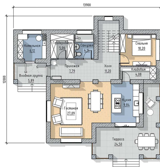
План 1 этаж
