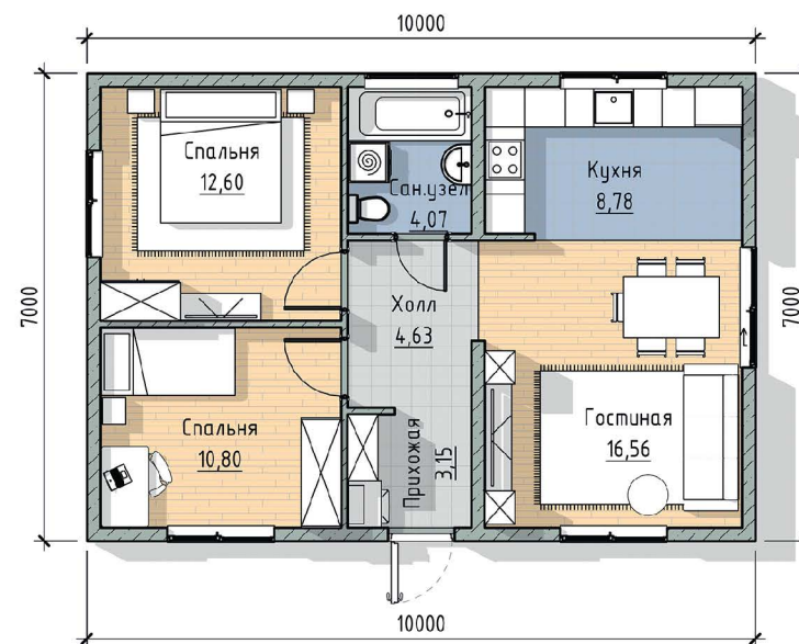
План
