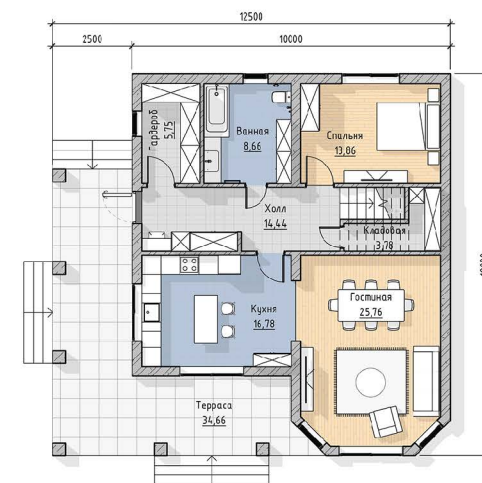
План 2 этаж
