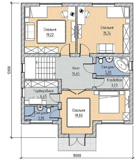
План 2 этаж
