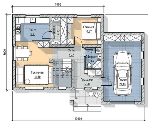
План 1 этаж
