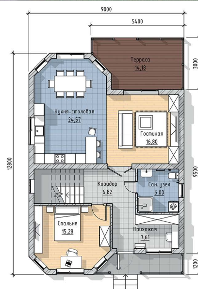
План 1 этаж
