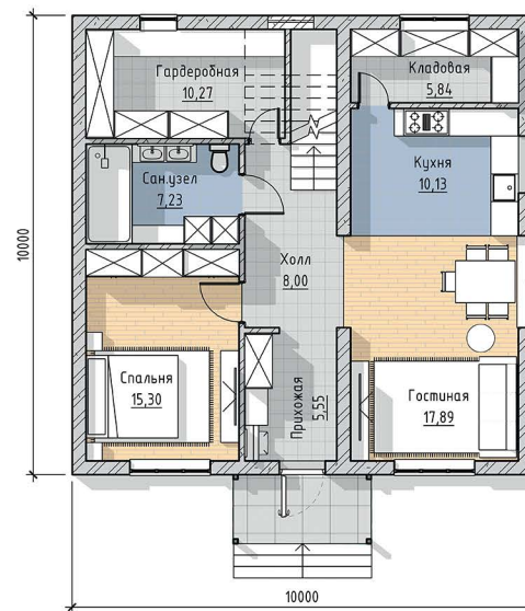
План 1 этаж
