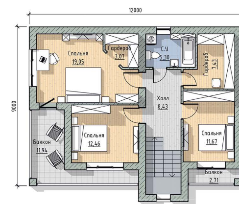
План 2 этаж
