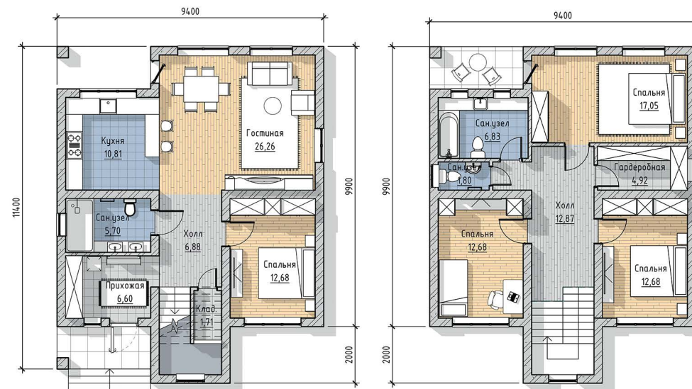
План 1 этаж
