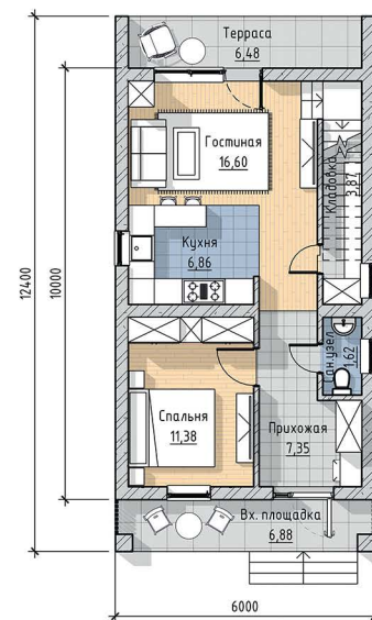
План 1 этаж
